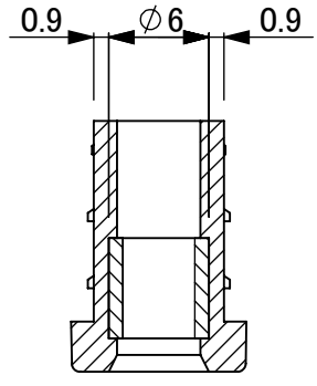
断面図 B-B
