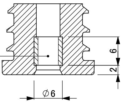
断面図 A-A
