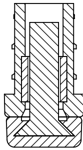
断面図 Z-Z
